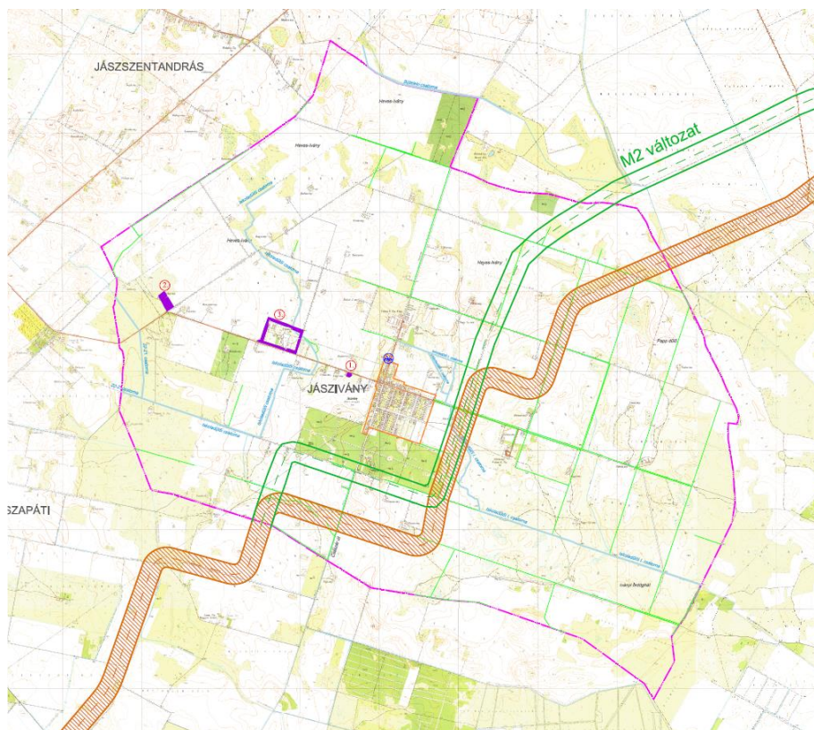
Jászági főcsatorna zagyvai ág nyomvonalváltozatok (KÖTIVIZIG adatszolgáltatás)
